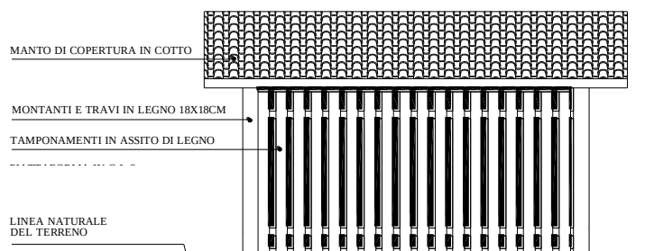
PROSPETTO LATERALE
